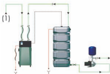
BWT PERMAQ® Pico Réservoir d'eau pure Système de surpression
