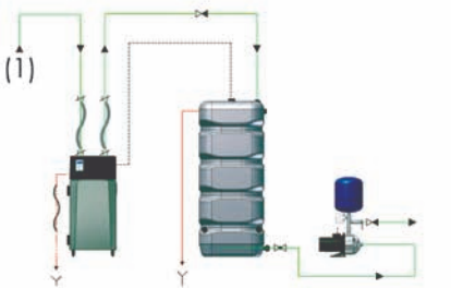
BWT PERMAQ® Reinwassertank Pico Druckerhöhungsanlage
